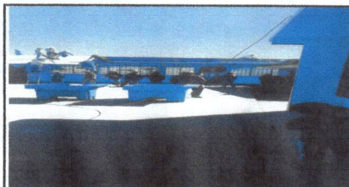
Foto 4: Modulos de aulas 3 y 4: desinstalación de lámina existente; sustitución de lámina por lámina troquelada aluzinc calibre 26 e instalación de canales.
